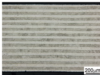
■開発した複層鋼板の断面観察（光学顕微鏡）
