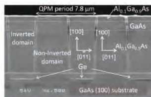
周期空間反転 GaAs/AlGaAs 波長変換 デバイス
