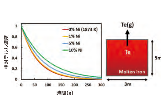
■テルル (Te) (快削鋼添加元素) の溶鉄からの蒸発速度と合金元素 (ニッケル, Ni) 濃度の影響
