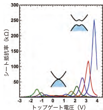
■2層グラフェンのトランジスタ動作
