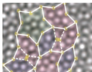
ボロン系準結晶の透過型電子顕微鏡写真
