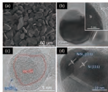
■プラズマスプレーによる様々なナノ構造 Si 粒子を負極として利用した電池は高い充放電サイクル容量特性を示す
