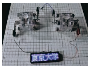
鉄族金属硫化物と炭素の複合材料を触媒に用いた 亜鉛空気電池
