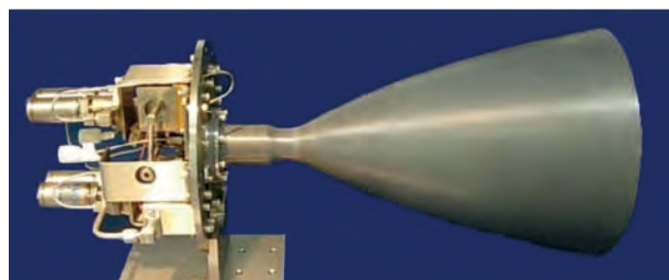
世界初のセラミック製スラスタ（金星探査機「あかつき」搭載）
