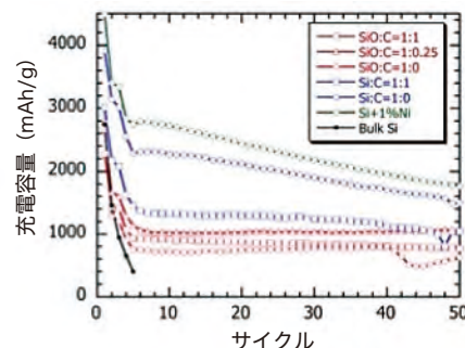
■プラズマスプレーによる様々なナノ構造 Si 粒子を負極として利用した電池は高い充放電サイクル容量特性を示す
