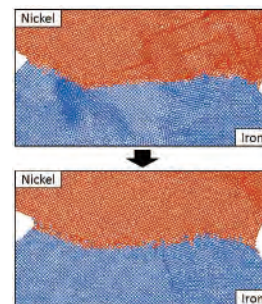
■異種材料間の界面形成過程の 経時変化シミュレーション
