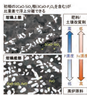
■製鋼スラグの冷却速度制御による高付加価値化
